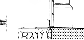
lower door stop, new
